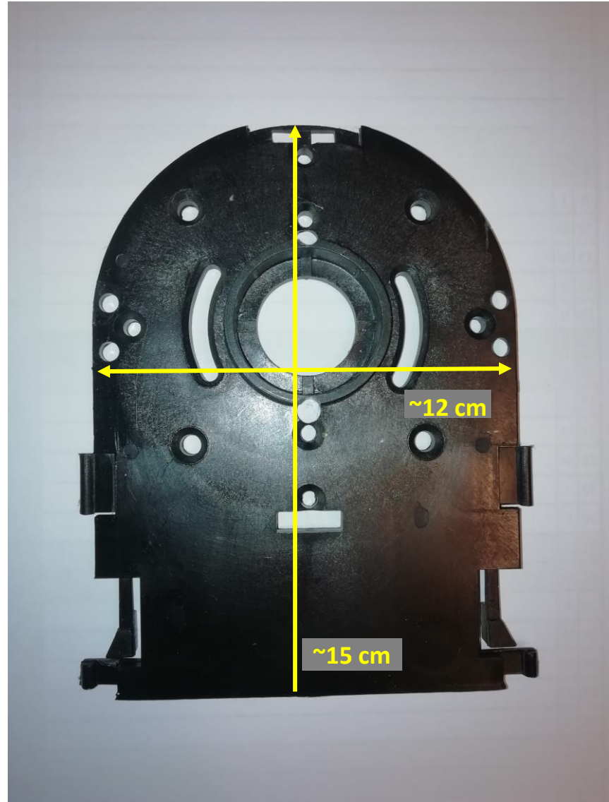
Côté sans moteur sans volet
