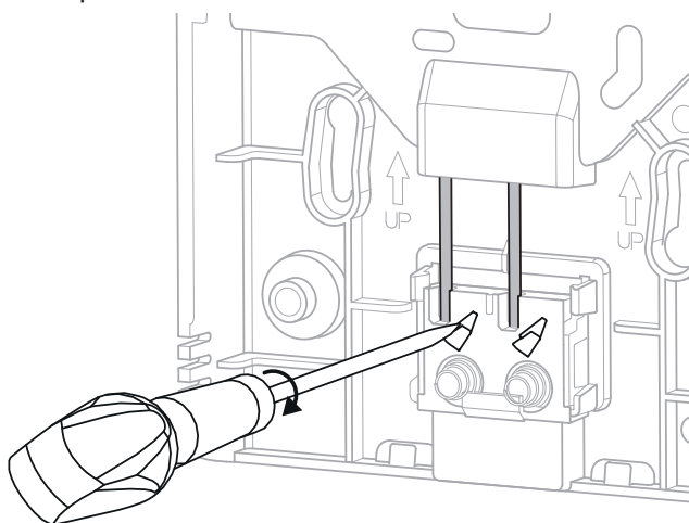
fig. 5 - Déconnexion des câbles
