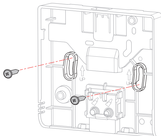
fig. 6 - Fixation au mur
