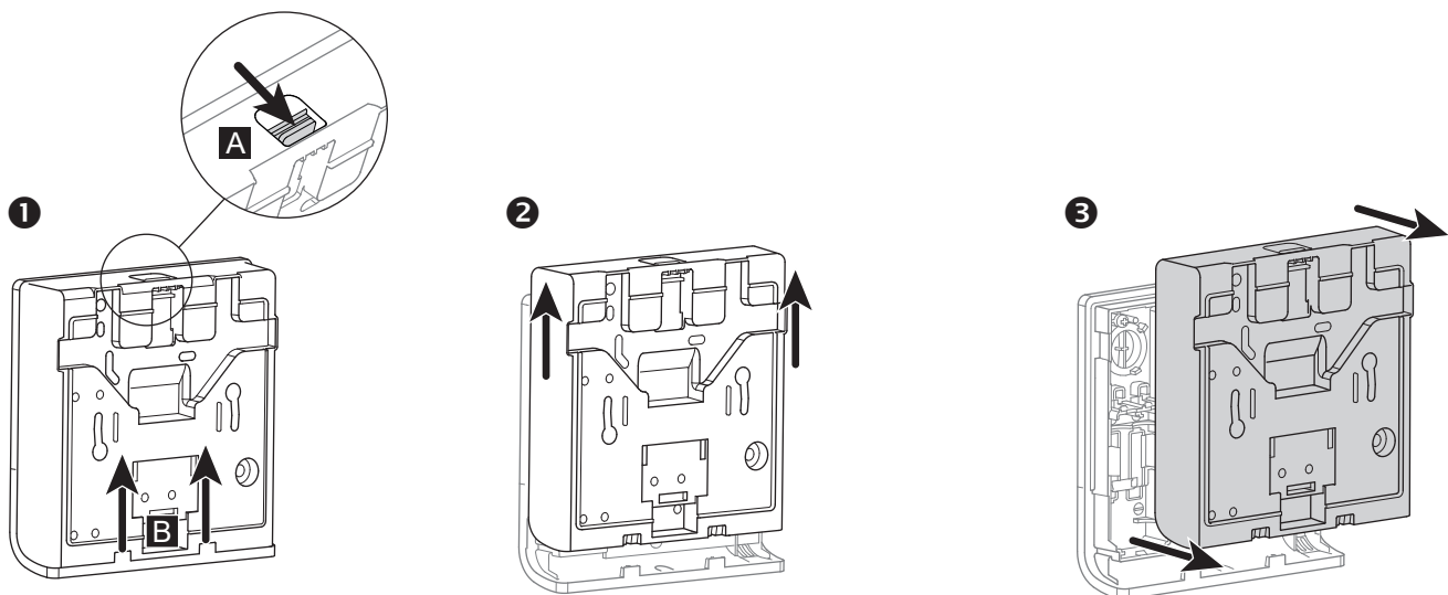
fig. 2 - Ouverture de la sonde
