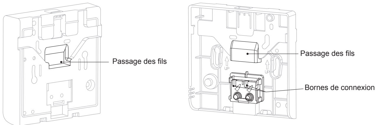
fig. 4 - Connexion des câbles
