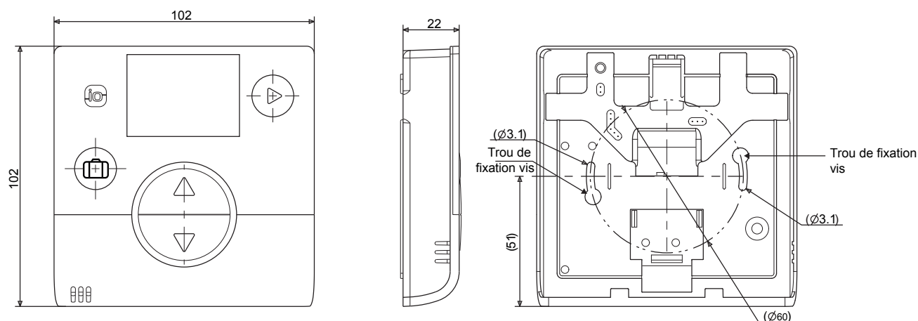
fig. 1 - Dimensions en mm
